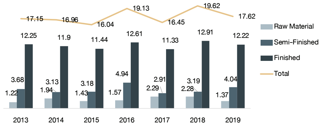
กราฟแสดงปริมาณการนำเข้าผลิตภัณฑ์หลักของไทย (หน่วย: ล้านตัน) ที่มา : กรมศุลกากร ประมวลผลโดยสถาบันเหล็กและเหล็กกล้าแห่งประเทศไทย
