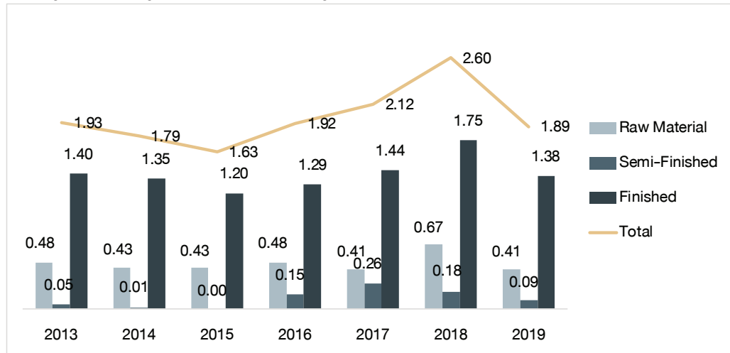
กราฟแสดงปริมาณการนำเข้าผลิตภัณฑ์เหล็กของไทย (หน่วย: ล้านตัน) ที่มา : กรมศุลกากร ประมวลผลโดยสถาบันเหล็กและเหล็กกล้าแห่งประเทศไทย
